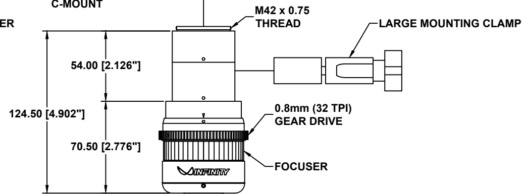
T-2 ADAPTER
